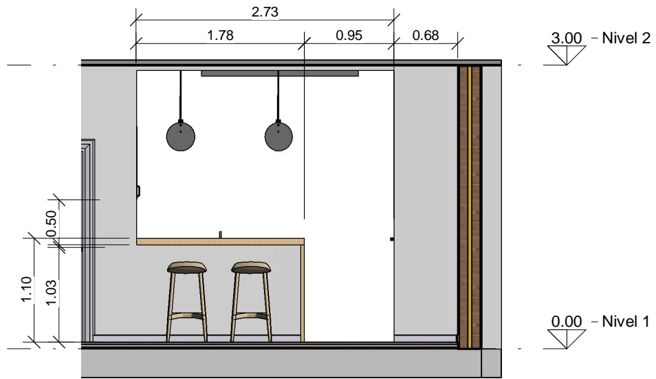
1 SECCIÓN COCINA A105 REFORMA 1
