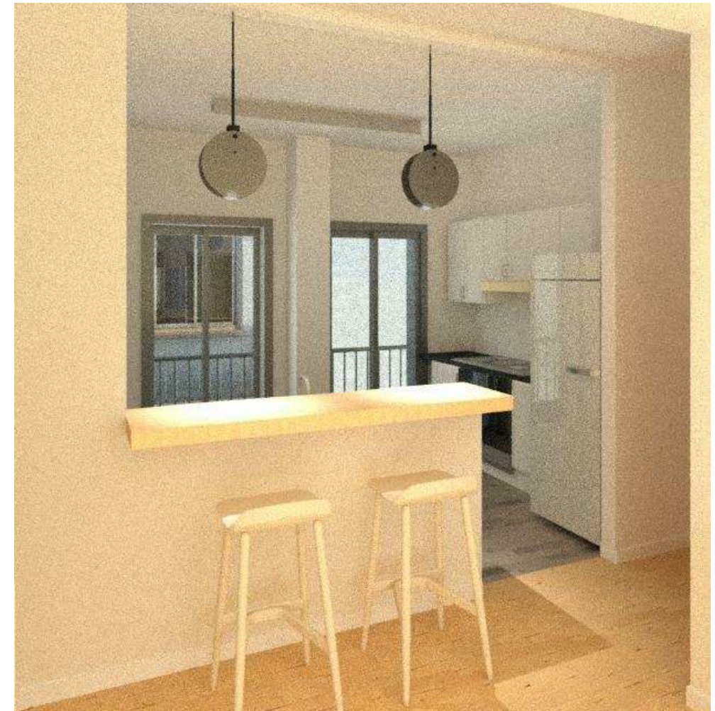
4 Vista 3D cocina reforma 1 A105 1:1
