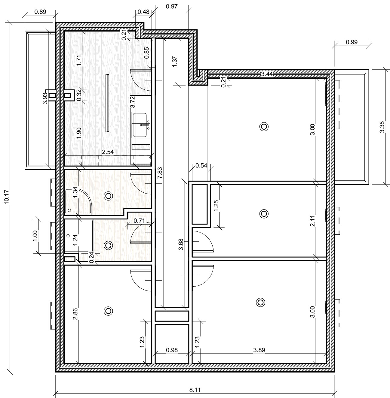
1 Planta estado inicial A107 1 : 60
