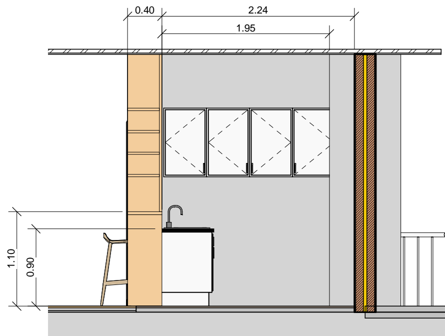
4 sección frontal 2.2 A108 1:40
