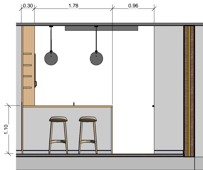
1 Detalle. Opción 2.2 A108 1:37
